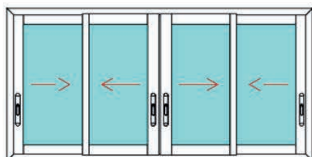
Coulissant 2 rails et 4 vantaux face à face
